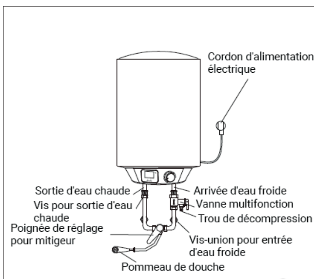
CONNEXION TYPIQUE À UNE SEULE SORTIE (Fig.3)
