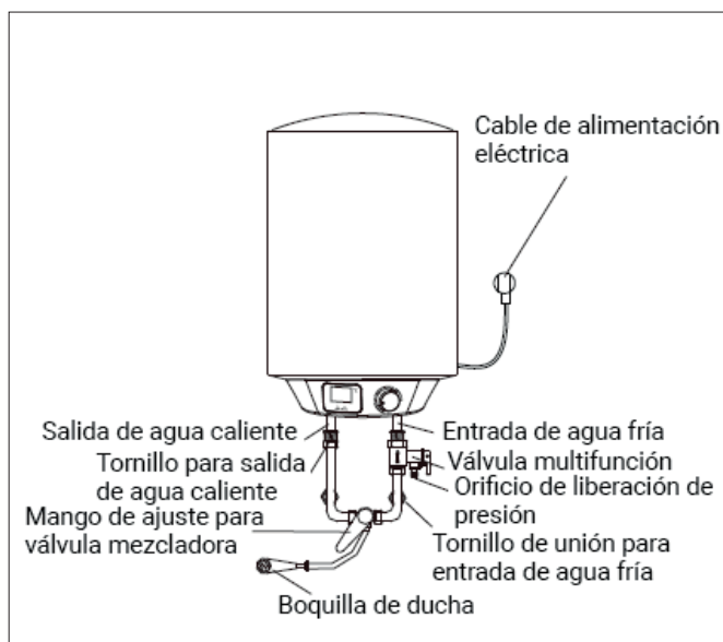
CONEXIÓN TÍPICA DE SALIDA ÚNICA (Fig.3)
