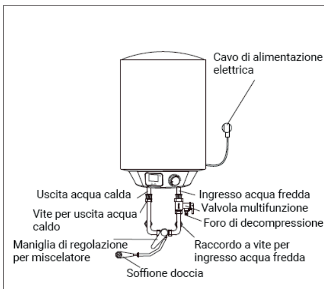
TIPICO COLLEGAMENTO A USCITA SINGOLA (Fig.3)
