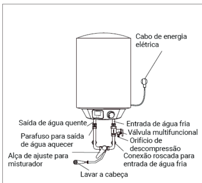
LIGAÇÃO TÍPICA DE SAÍDA ÚNICA (Fig.3)
