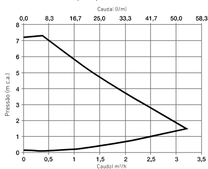
Curva do circulador incluído nos modelos GT, GTF, GTA e GTAF
